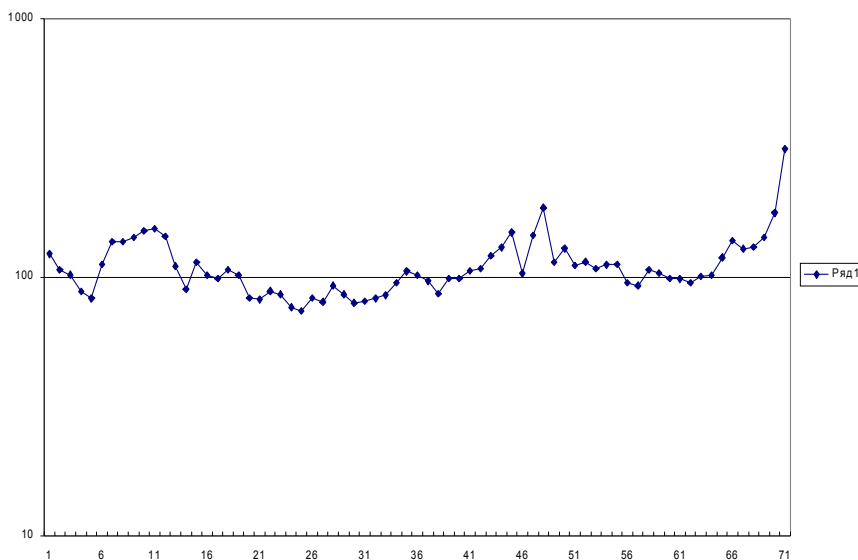
Рис. 2. Геофизический профиль вдоль внутреннего вала Малобыковского городища-1 в направлении с запада на восток
